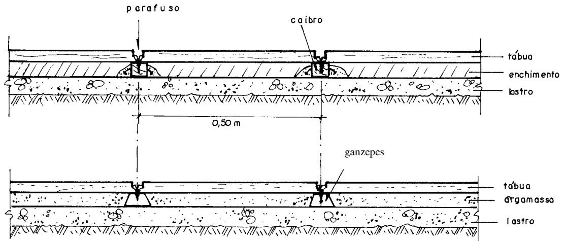
Figura 8.12 - Fixação das tábuas com parafusos sobre caibros ou ganzeipes
